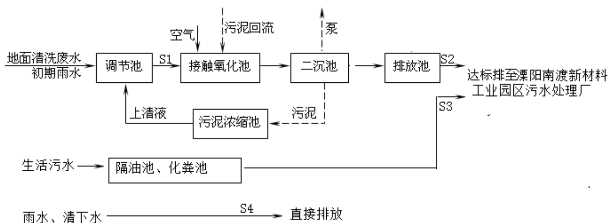
图 4-1 污水处理流程图
