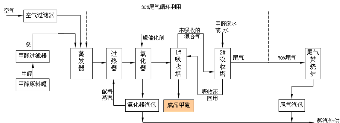
图 3-2 甲醛工艺流程简图
