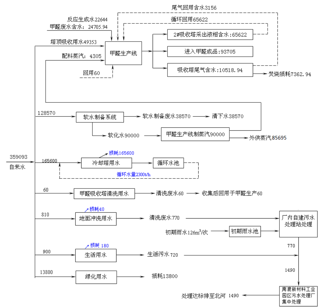
图 3-1 甲醛厂区用水平衡图（单位：t/a）
