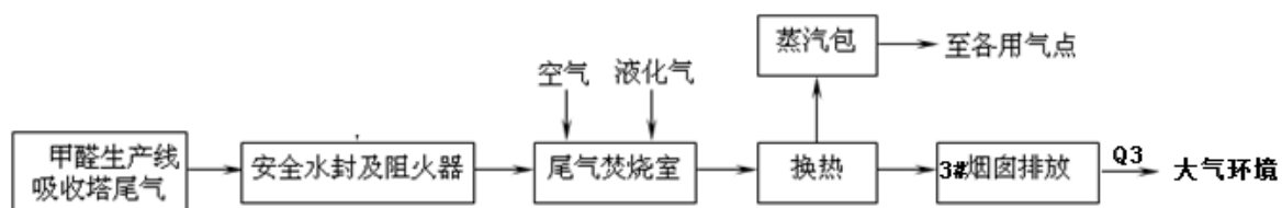
图 4-3 甲醛吸收塔尾气焚烧处理流程
